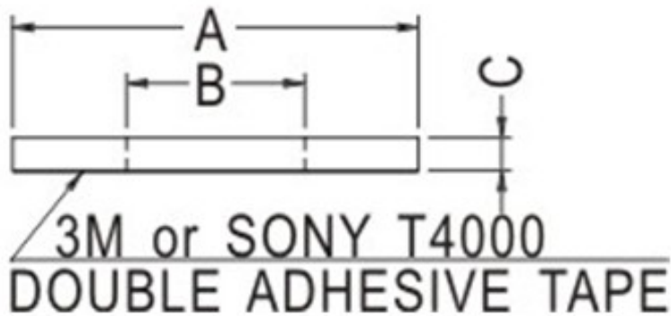
RNWF-8 结构图
