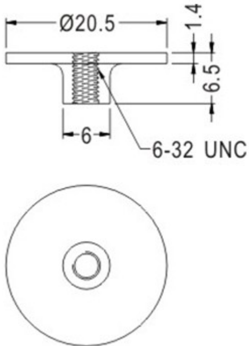
LTRMH-1 结构图
