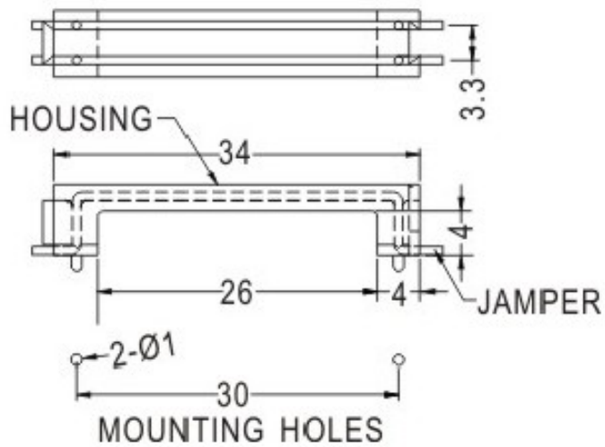
JUP-1 结构图
