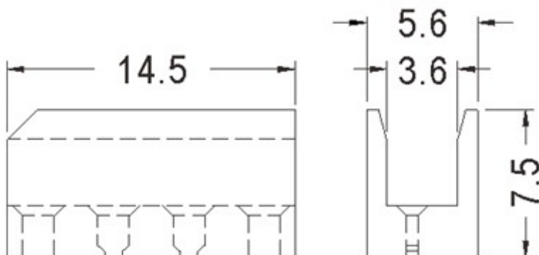
LBG03 结构图
