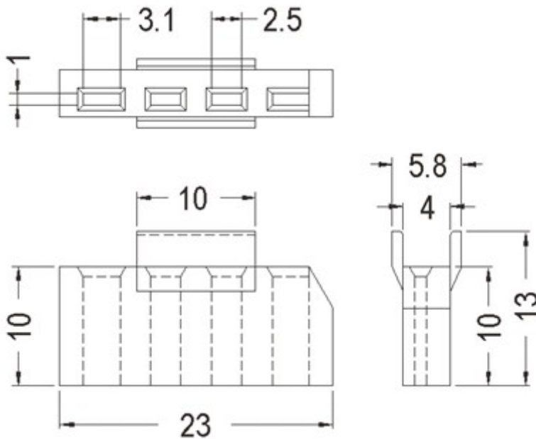
LBG04 结构图
