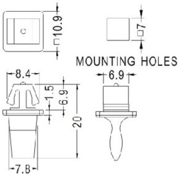
DDK-7 结构图
