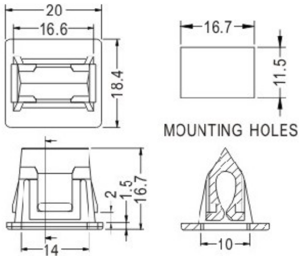
DDK-6 结构图
