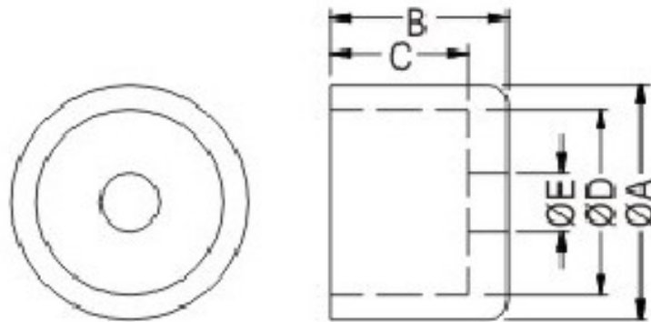
MC-04 结构图
