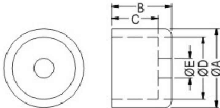
MC-02 结构图
