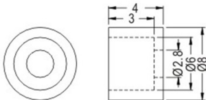
MC-08 结构图
