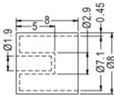
MC-05 结构图
