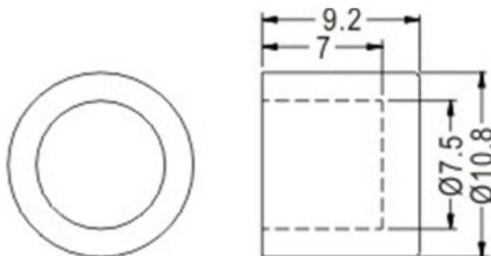
MC-07 结构图
