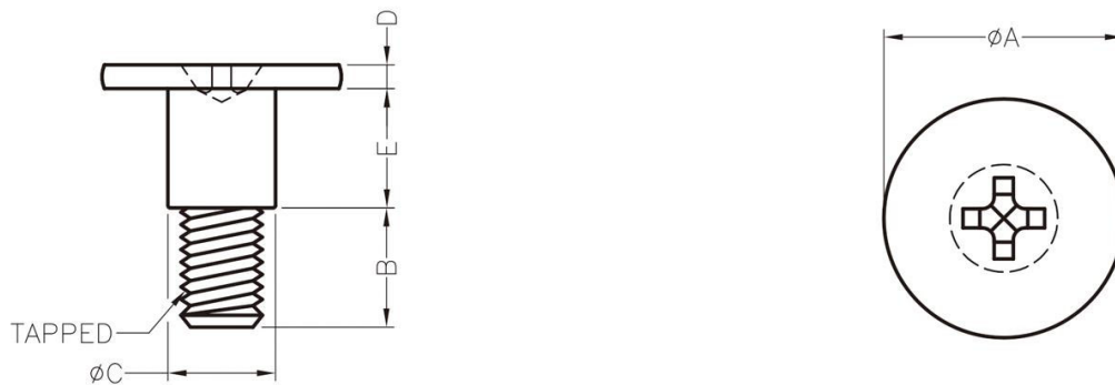
GPEK-08 结构图
