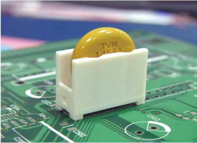
PAHO-034 结构图
