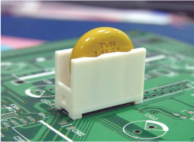
PAHO-035 结构图
