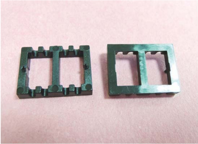
PAHO-057 结构图
