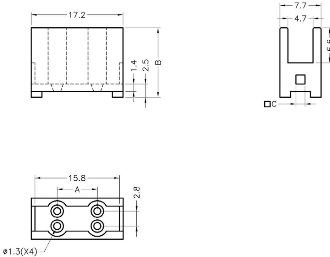
PAHO-037 结构图
