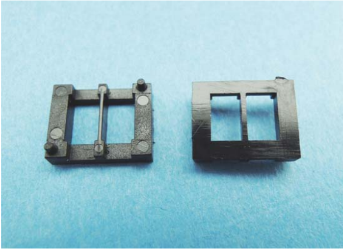
PAHO-056 结构图
