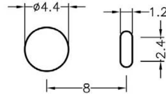
HOLE IN P.C.B
