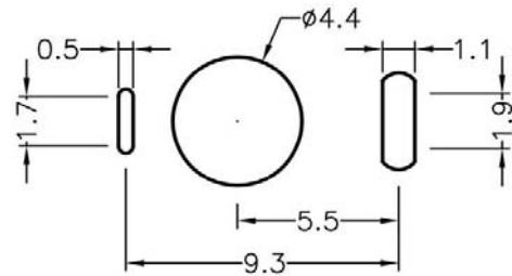
HOLE IN P.C.B
