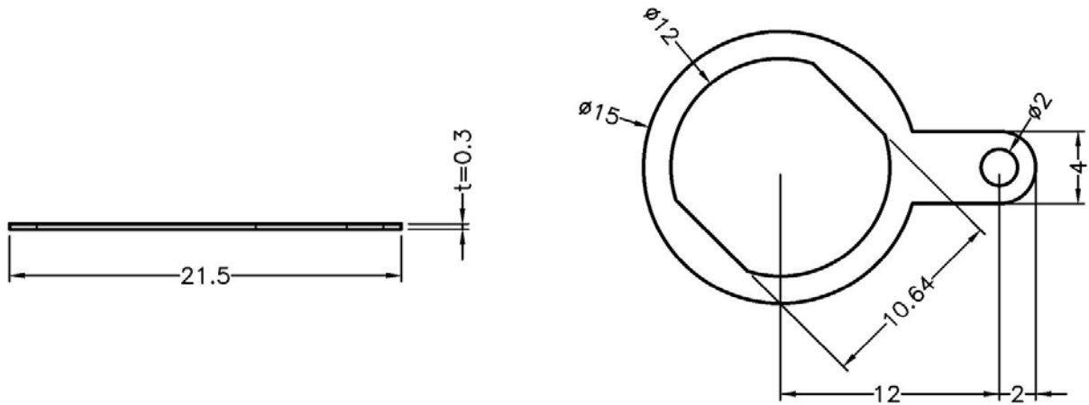
GNT E-21 结构图
