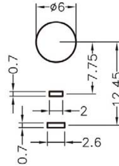
HOLE IN P.C.B
