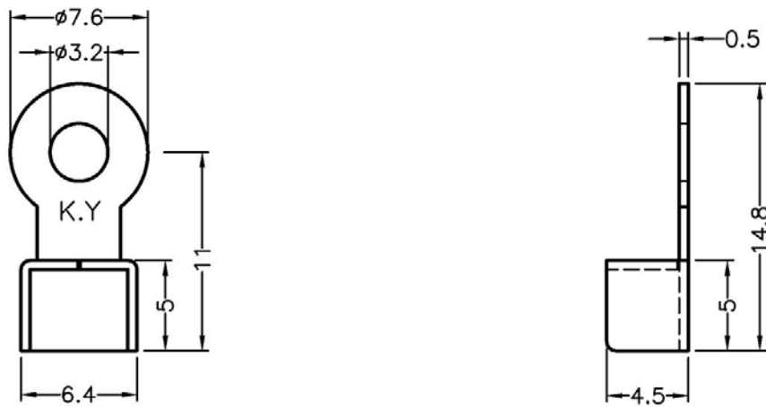
GNTE-22 结构图
