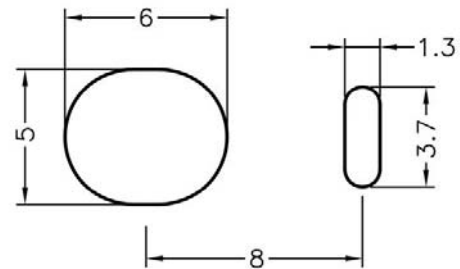
HOLE IN P.C.B
