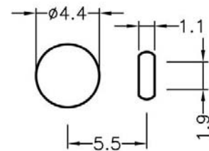
HOLE IN P.C.B
