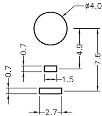
HOLE IN P.C.B
