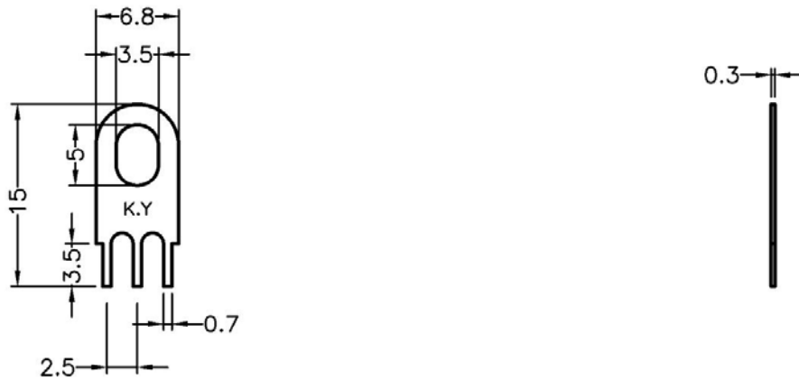
GNT E-25 结构图
