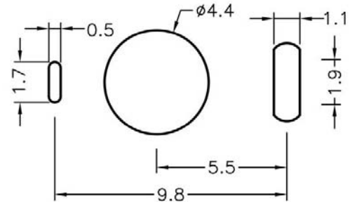
HOLE IN P.C.B
