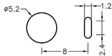
HOLE IN P.C.B
