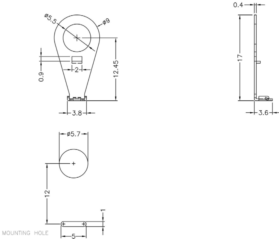
GNT E-45 结构图
