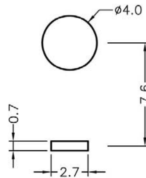
HOLE IN P.C.B
