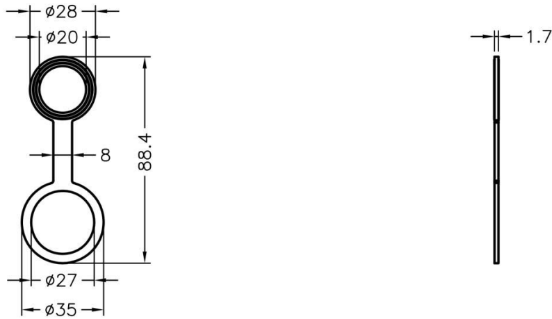
TF-L1 结构图
