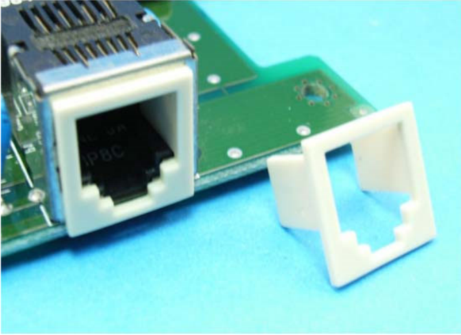
DZGR-03 结构图
