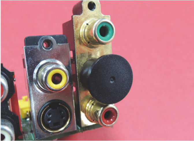
DZGR-09 结构图
