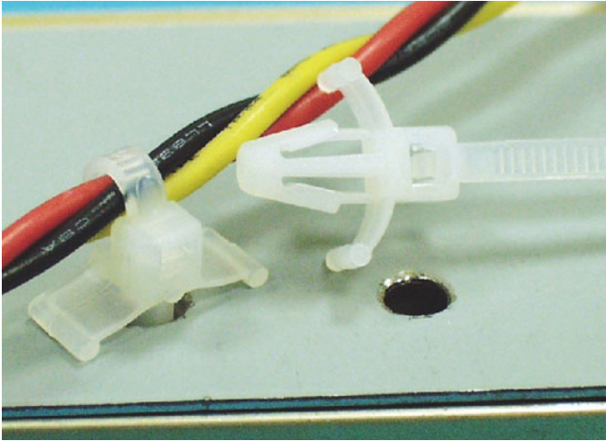
DYS-008 结构图
