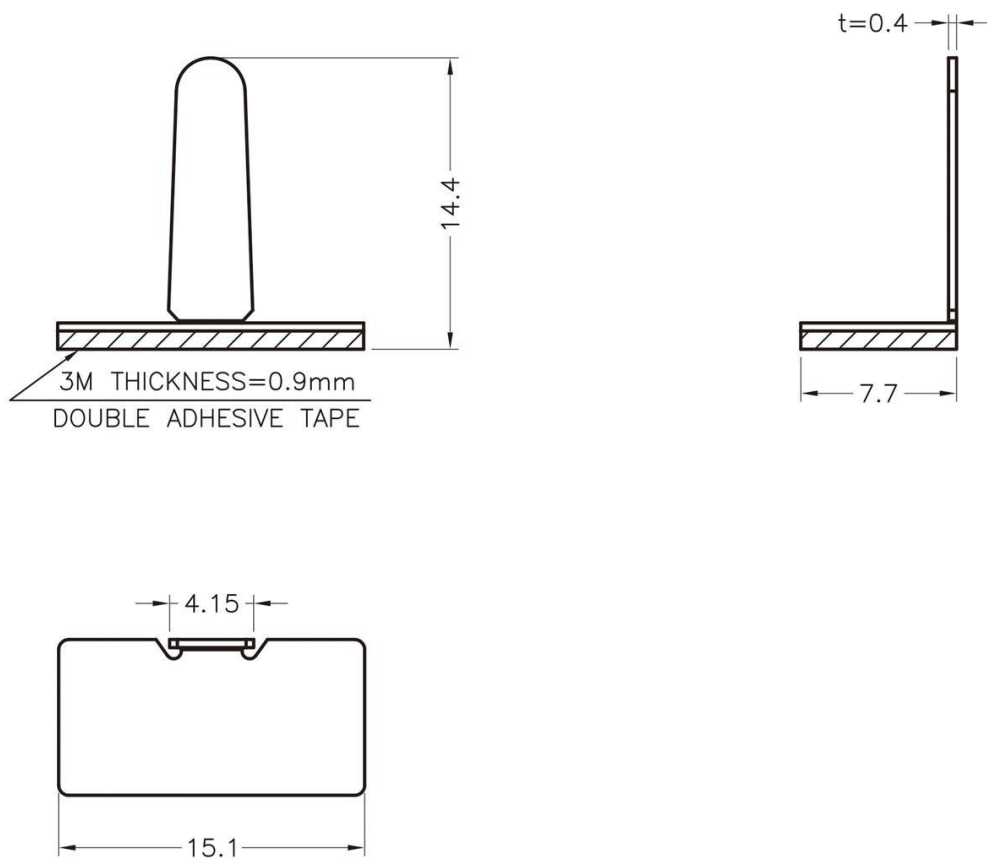
DXG-3 结构图
