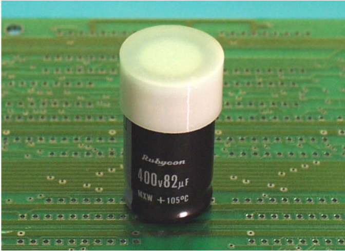
BCCT-02 结构图
