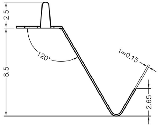
TRNK-002 结构图
